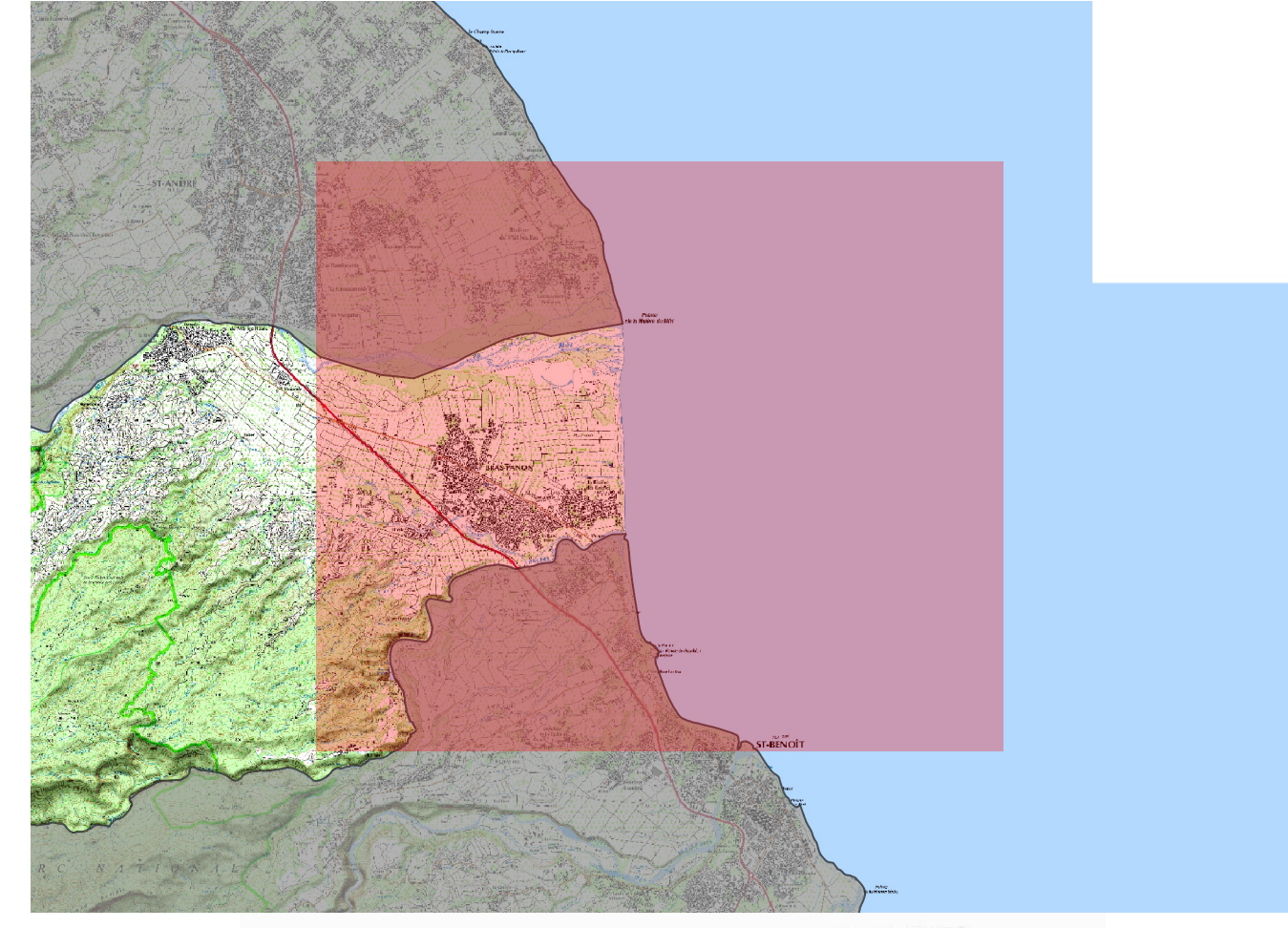
Carte de synthèse de l'évolution historique du trait de côte
